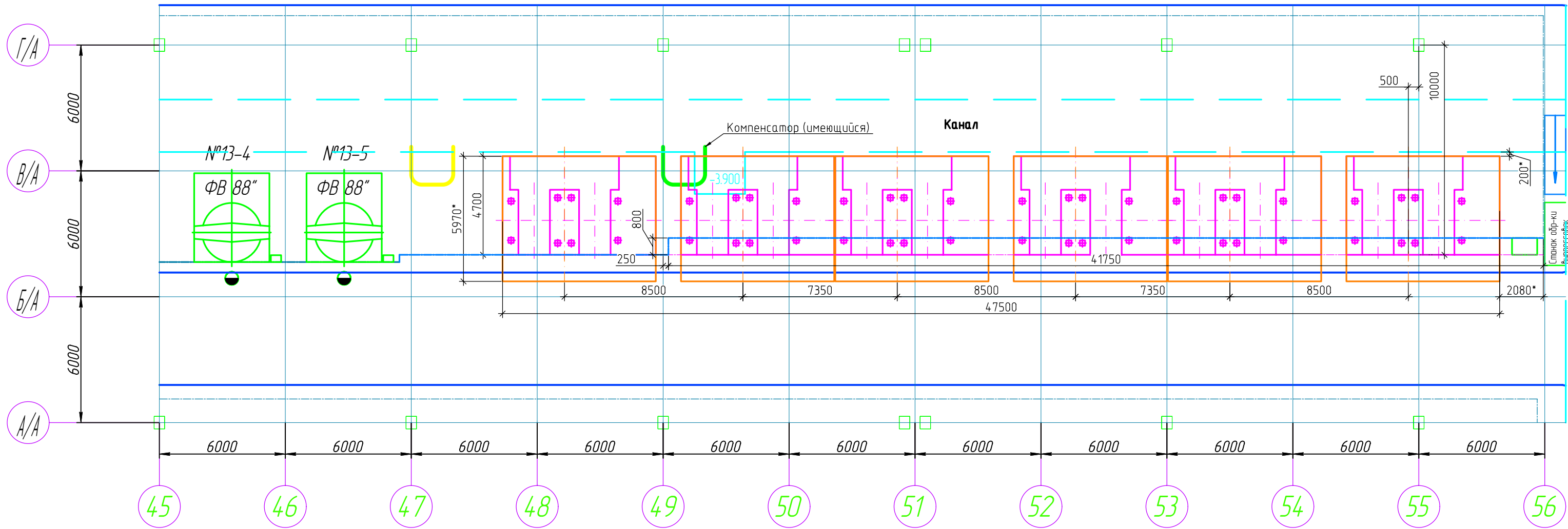
Фундамент Ф/В 13 ряд
