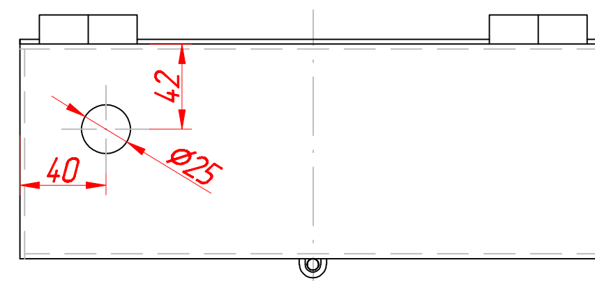
Вид С
